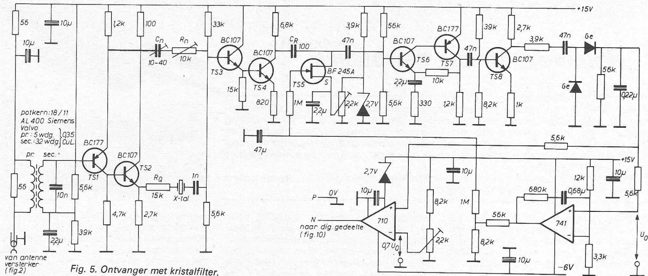
Fig. 5. Ontvanger met kristalfilter.
