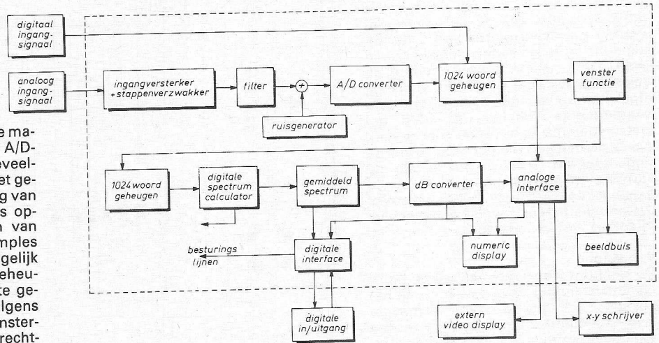
Fig. 7. Blokschema van de spectrum-analyser.
