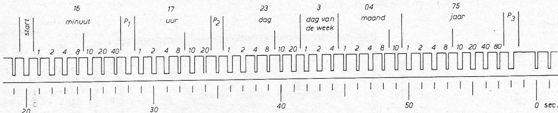
Fig. 1. Pulsvolgorde diagram van het uitgezonden signaal.
