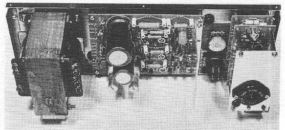
Afb. 3 Achterpaneel van de enkelvoudige oscilloscoop. In het midden de voedingsprint.
