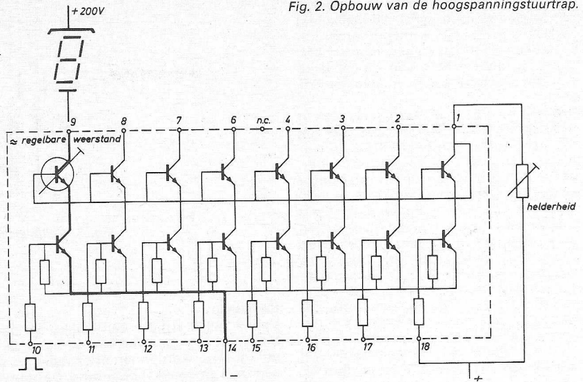
Fig. 2. Opbouw van de hoogspanningstuurtrap.
