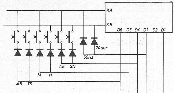
Fig. 3. Gelijktzercircuit.
