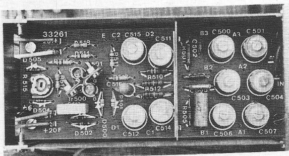
Afb. 2 Verzwakkerenheid, duidelijk is te zien dat de FET's in hetzelfde koellichaam zijn gemonteerd.
