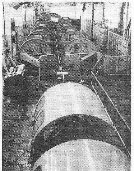
Voor het torsievrij slaan van telefoonkabels en voor het vervaardigen van coaxkabels, ontwikkelde Krupp een nieuwe draadslagmachine. De maximale tordering bedraagt ongeveer 2%.
