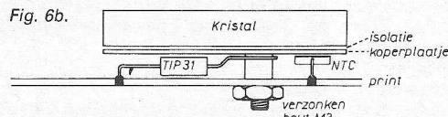
Fig. 6. Temperatuurstabilisatie van het kristal en de bevestigingsmethode.
